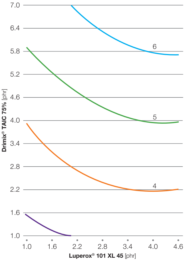
Modulus 100 % [MPa]
